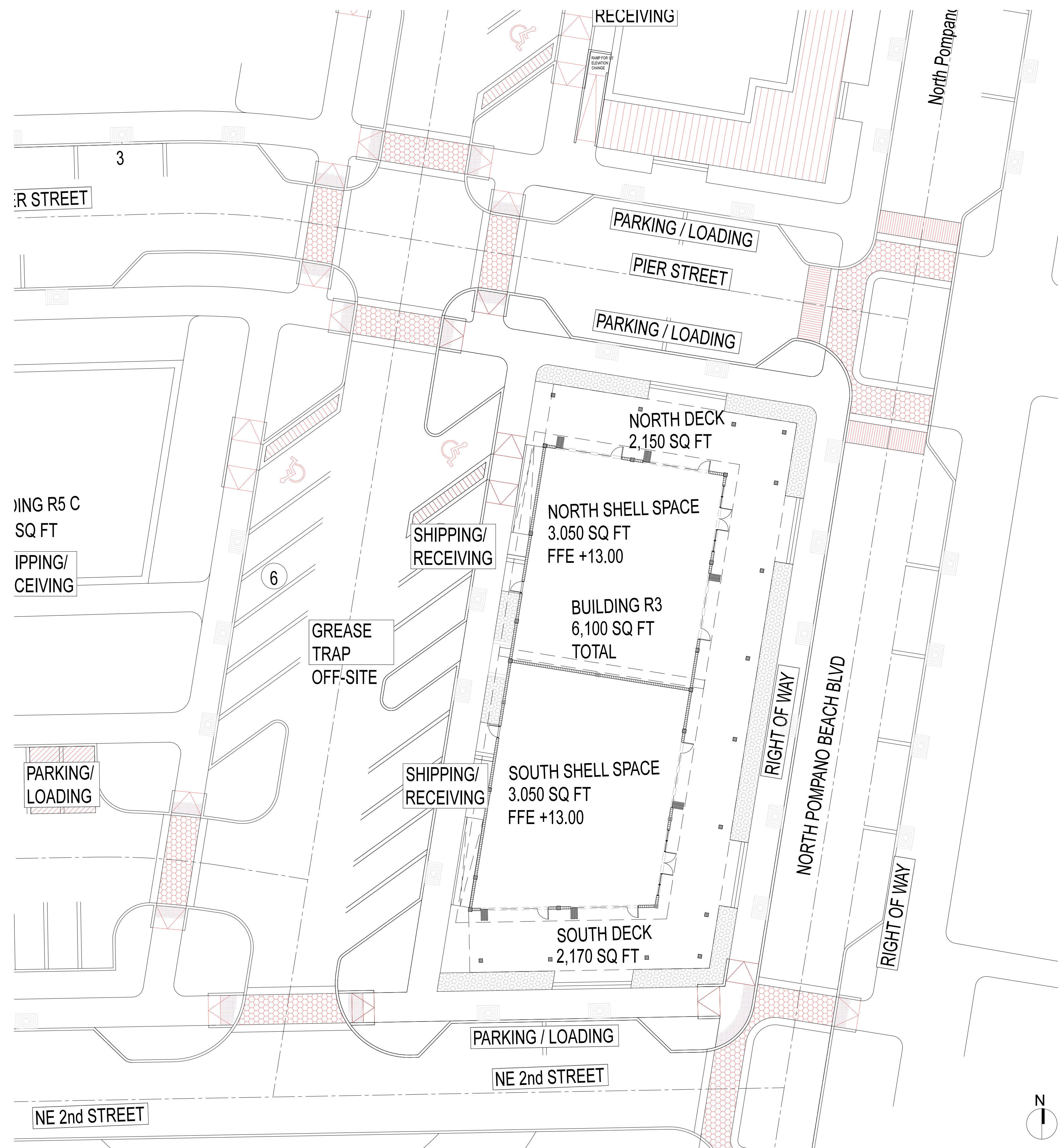
01 SITE PLAN SCALE: 1/16"=1'-0"
